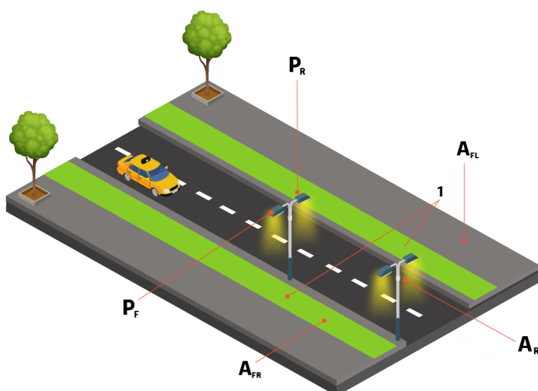
Figura 3.3.1.8. a. Ejemplo perfil vía para calculo PDI(Dp) y AEI(DE). (Fuente propia)
